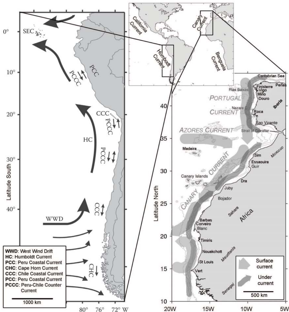
FIG. 1.2 – Présentation des régions étudiées. À gauche, le système d'upwelling du Courant de Humboldt (SCH) (d'après Thiel et al. , 2007) et à droite le système d'upwelling du Courant des Canaries (SCC) (d'après Aristegui et al. , 2006).
