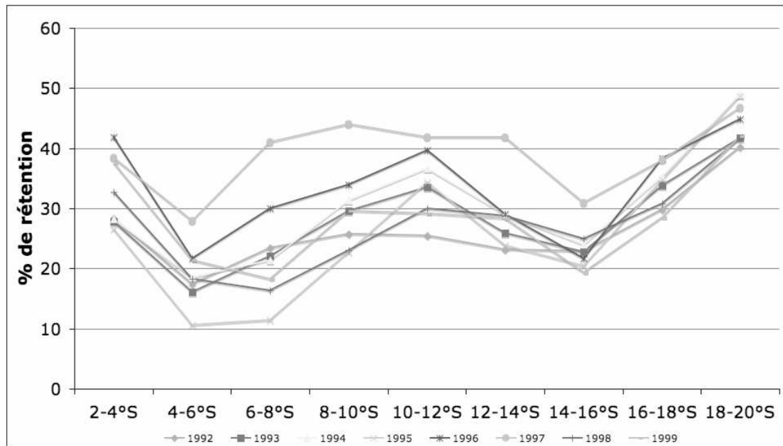
FIG. 2.13 – Effet de l'interaction latitude x année sur le pourcentage de rétention.
