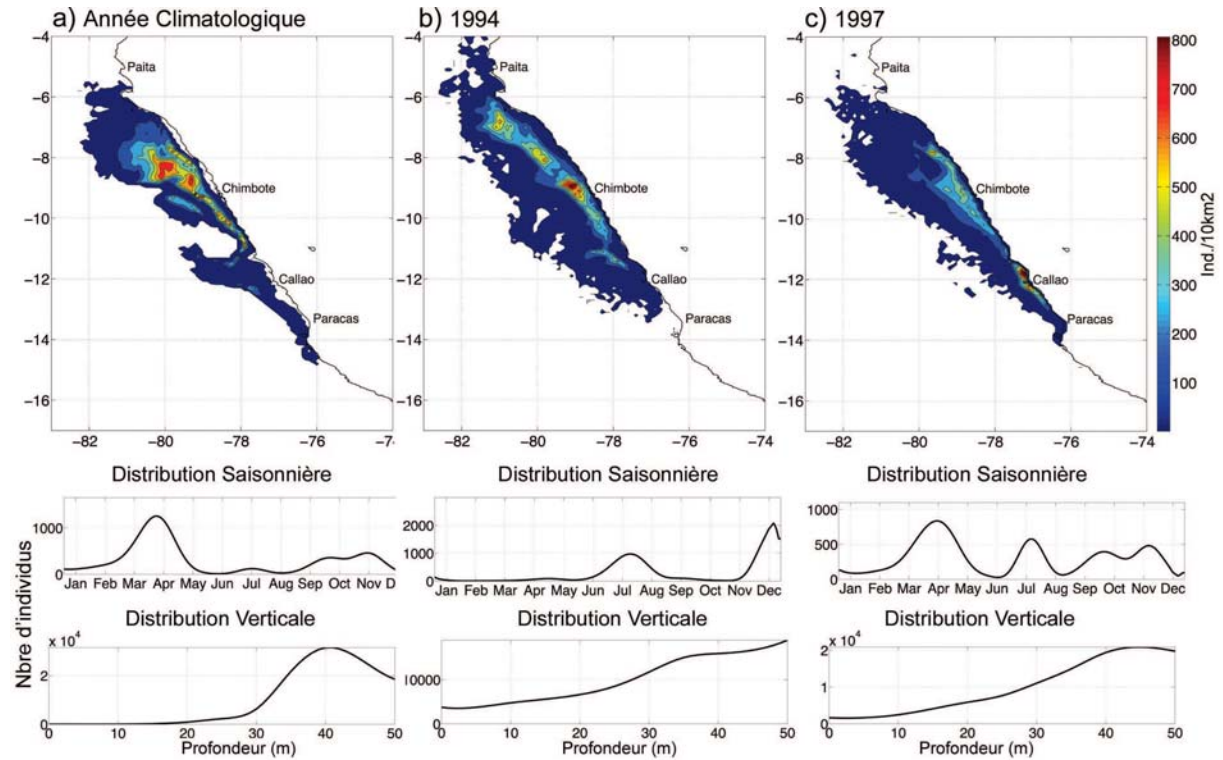
FIG. 4.7 – Simulation 3 : Pattern de ponte horizontal, saisonnier et vertical émergeant pour une année climatologique (a) et deux années issue d'un forçage interannuel correspondant à 1994 (b) et 1997 (c).
